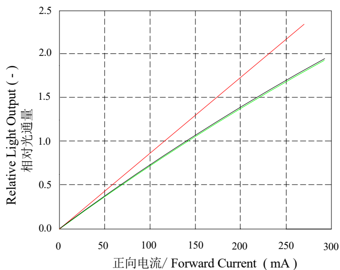
Forward Current vs. Light Output (Ta=25°C) 正向电流与光通量曲线图
