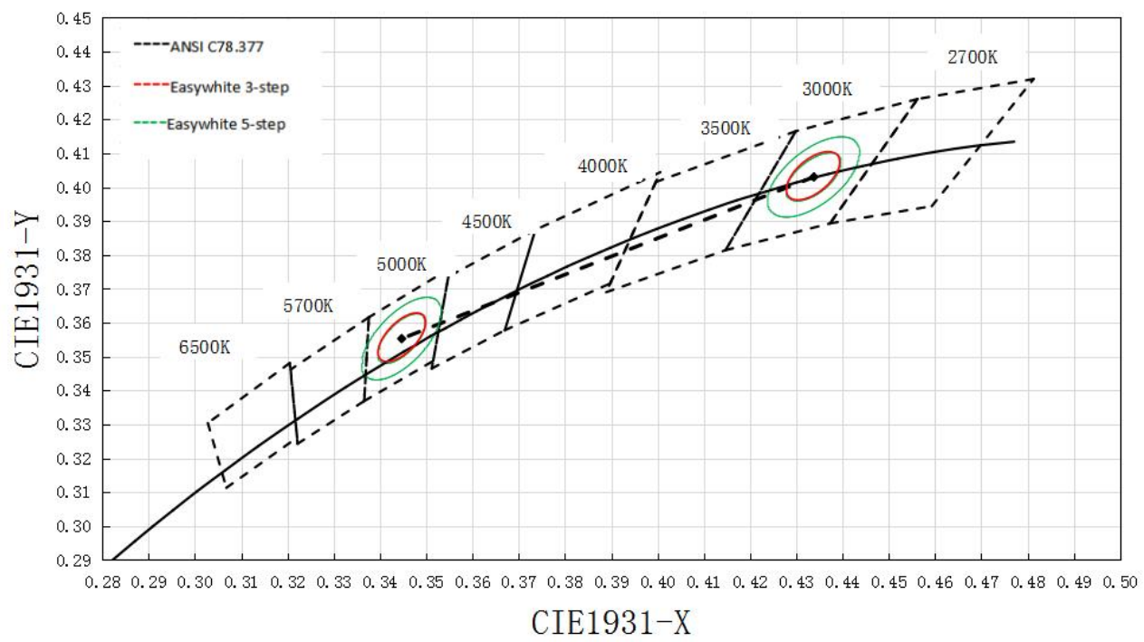
CIE(X, Y)坐标 CIE coordinates (X, Y)
