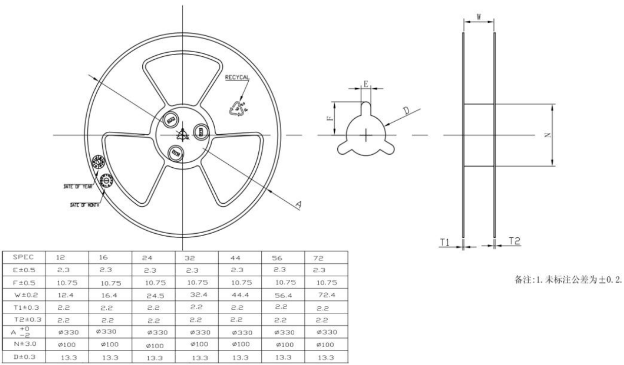
铝箔袋标签 Aluminum foil ba 卷盘尺寸/Reel Dimensions (单位:毫米 Units:mm)
