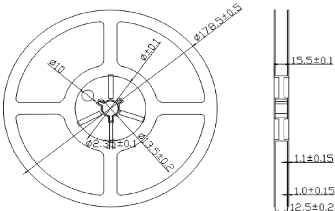
铝箔袋标签 Aluminum foil ba 卷盘尺寸/Reel Dimensions (单位:毫米 Units:mm)
