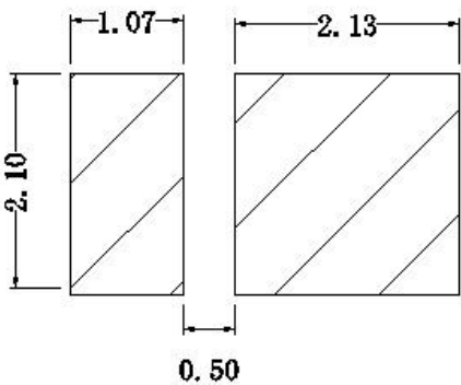
建议焊盘尺寸
