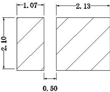
建议焊盘尺寸
