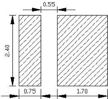
建议焊盘
