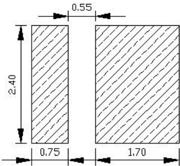
建议焊盘
