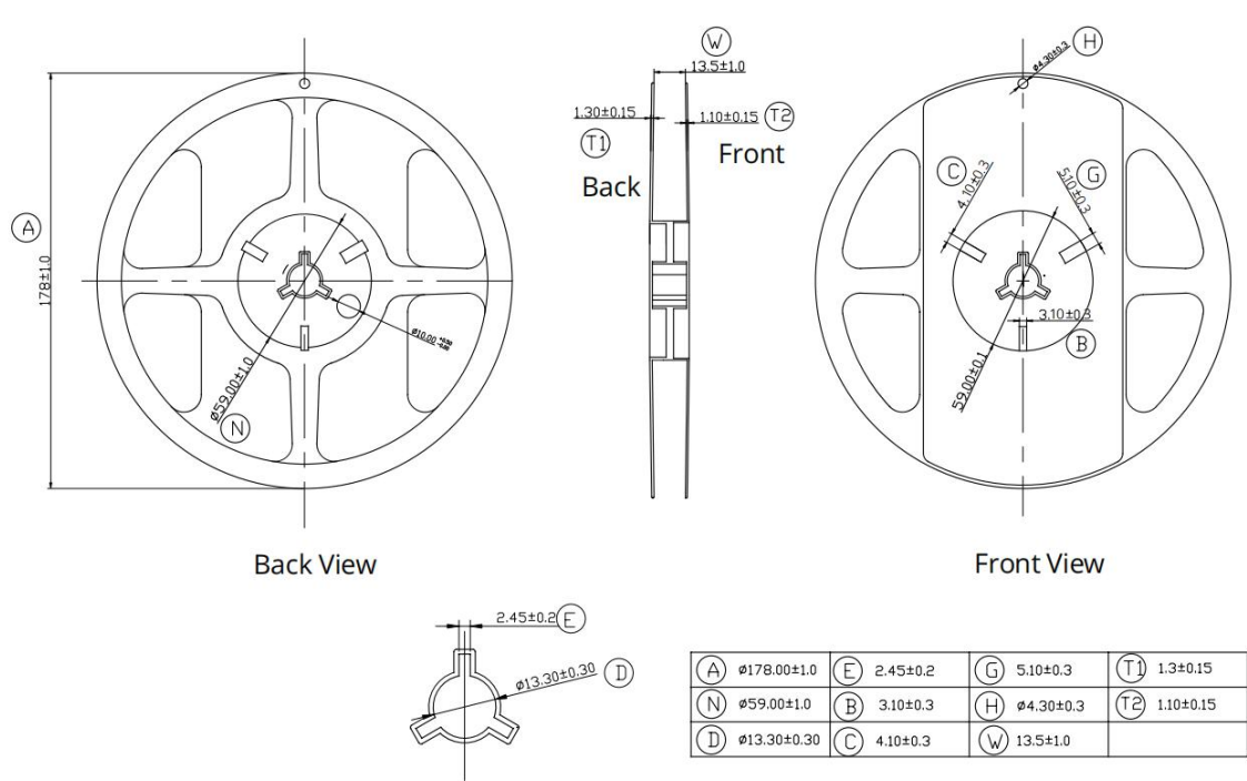
卷盘尺寸/Reel Dimensions (单位:毫米 Units:mm)
